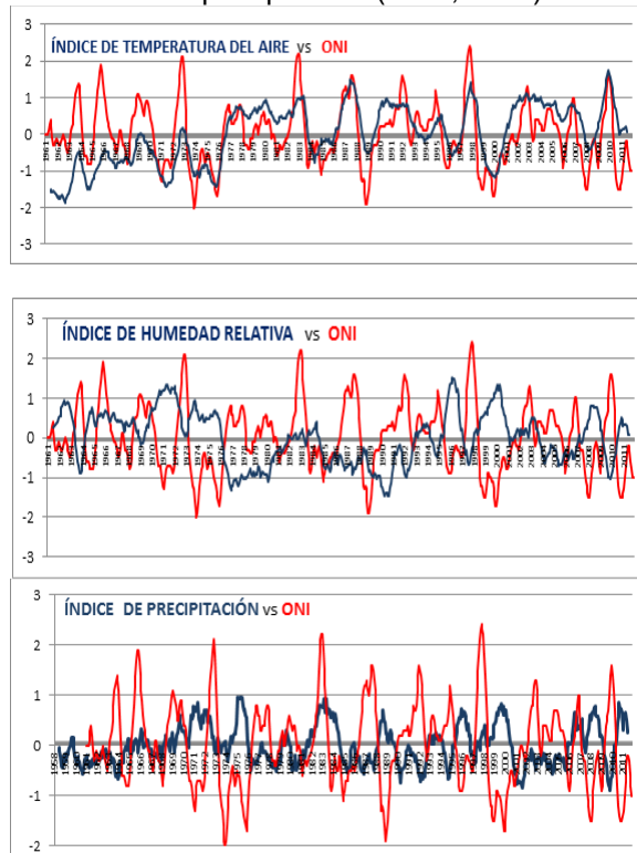
Figura 4. Secuencias de los índices de temperatura del aire, humedad relativa y de precipitación para la estación del Aeropuerto Mariscal Sucre de Quito comparado con el ONI en el período 1958-2011 (Fuente de datos: D.G.A.C.; NOAA)
