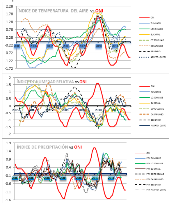
Figura 5. Índice de temperatura del aire, humedad relativa y precipitación de las estaciones DMQ vs ONI calculado para las siete estaciones analizadas para el período 2005-2011 (Fuente de datos REMMAQ; DGAC; NOAA)
