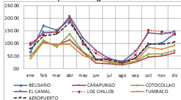
Figura 3. Ciclo anual de la precipitación en las estaciones del Distrito Metropolitano de Quito, construido para el período 2005-2011. (Fuente de datos: REMMAQ-D.G.A.C.)
